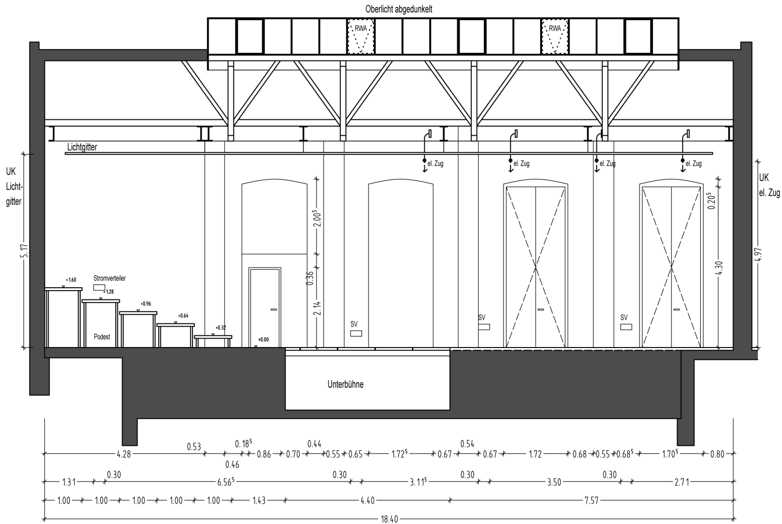
Längsschnitt M 1: 100
